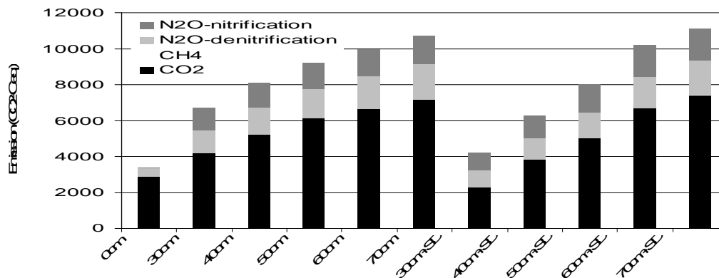
Figuur 2 Broeikasgasemissie afhankelijk van het slootpeil ( cm – maaiveld) met (SD) en zonder onderwaterdrains (Hendriks et al., 2008)
